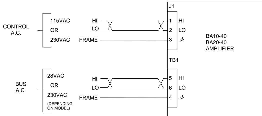
Figure 2-4. 40 Volt Option
